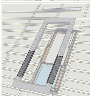
Beépítés kiegészítő elemmel GIL/GIU BFX WK34 0000
